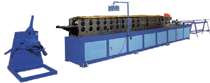
法蘭系統生產線
