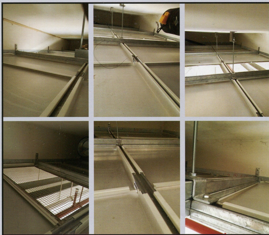
數據中心U槽天花頂層安裝實況
